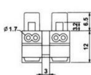
PA11-2 2 poles
