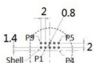
PCB板开孔尺寸
