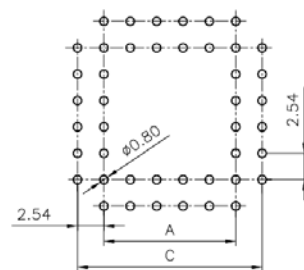
Рекомендации по отверстиям в печатной плате Допуск ±0.05 мм
