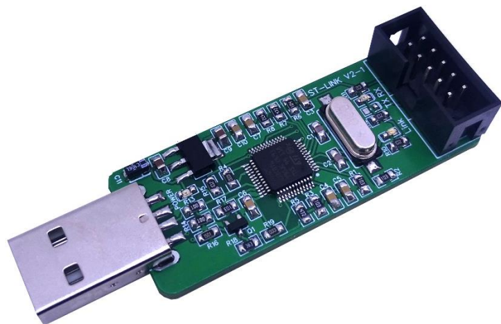
Набор для сборки программатора ST-Link 2.1
