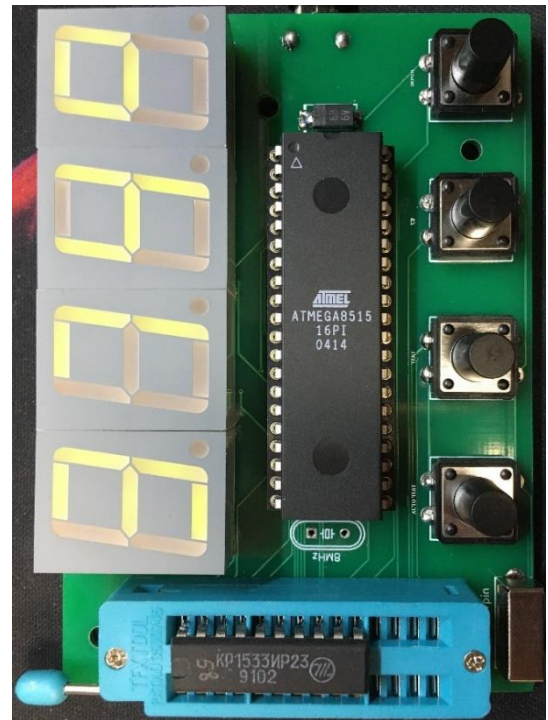
Тестер микросхем
