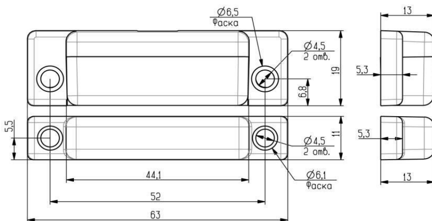
Рис.1. Габаритные и установочные размеры задающего и
