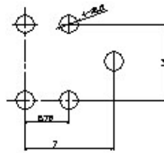
印制板布线 Recommended P.C.B layout
