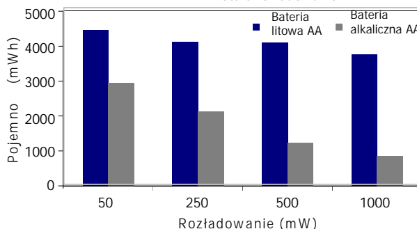
Temperatura pokojowa (21°C) Stałe rozładowanie
