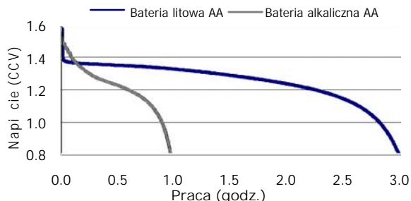
Charakterystyka stałego natężenia Typowe właściwości dla 1.0 V (21°C)
