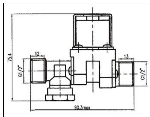
Рис.2. Установочные размеры.
