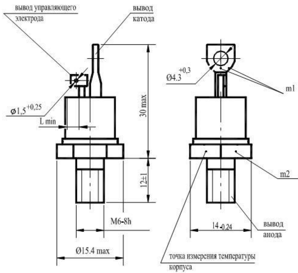
Тиристор Т122
