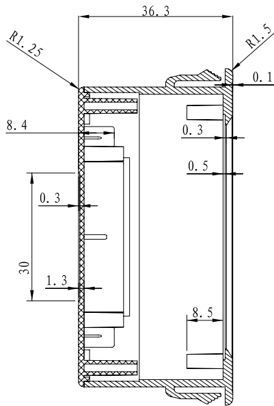
剖面 B-B
